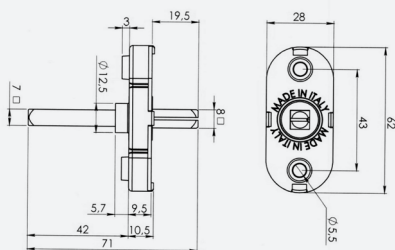
mechanika pre kľučku na eurookno
