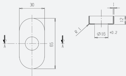
krytka mechaniky pre kľučku na eurookno
