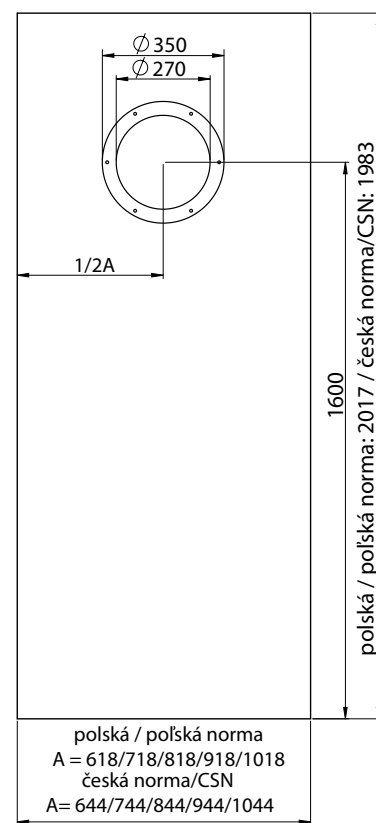
Konstrukce křídla Bulaj bezfalcový / Křídlová konštrukcia Bulaj bezfalcový
