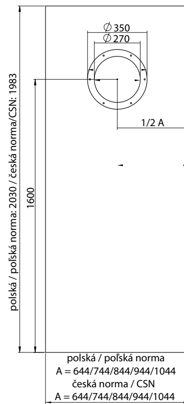
Konstrukce křídla Bulaj falcový / Křídlová konštrukcia Bulaj falcový
